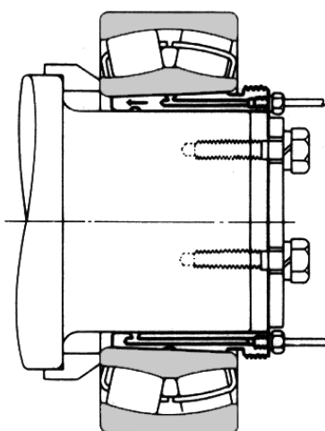
Установки при помощи специальной втулки и масла под давлением
